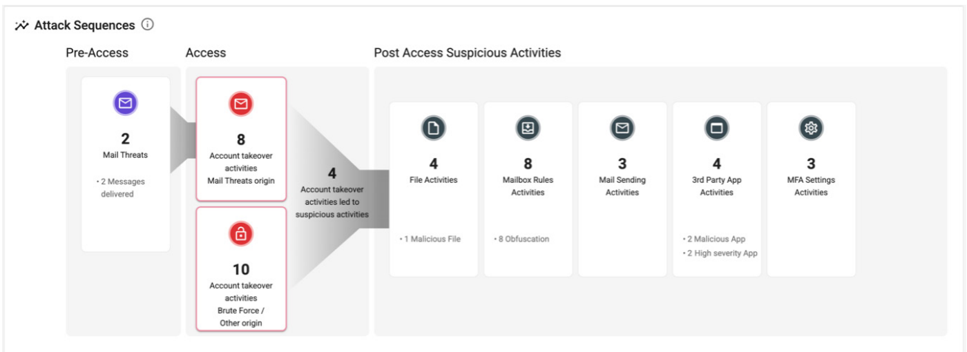
Figure 4. Proofpoint User Protection affiche les activités malveillantes antérieures et postérieures à l'accès pour les comptes affectés.
