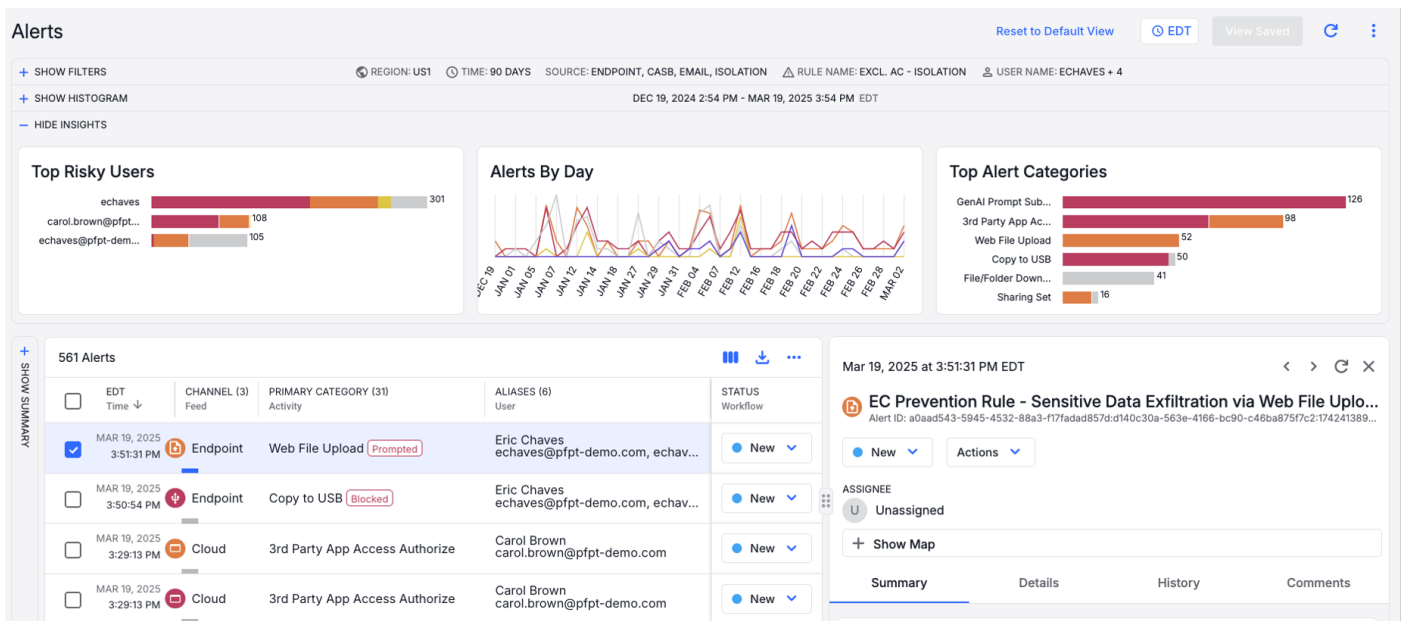
Figura 3. O Proofpoint Data Security Workbench simplifica o gerenciamento de alertas em e-mail, nuvem e endpoints sem a necessidade de múltiplos consoles. Neste exemplo, um analista filtra os alertas de um usuário específico. O dashboard mostra que o usuário fez upload de dados confidenciais para sua conta de e-mail corporativa e tentou copiar um arquivo para uma unidade USB antes de ser bloqueado.
