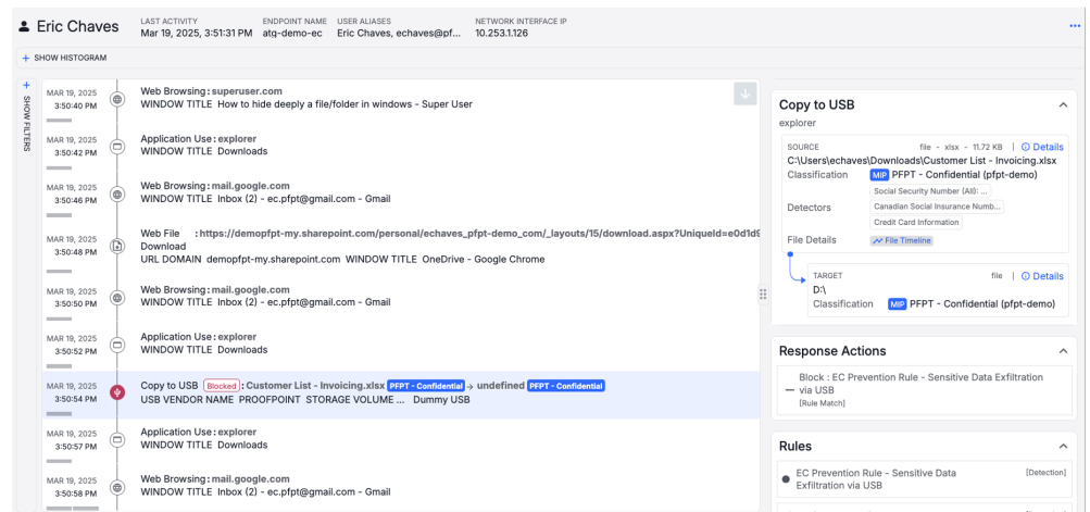
Figura 2. Nessa imagem de tela do console do Proofpoint Data Security Workbench, um usuário navega para um site chamado “Como esconder profundamente um arquivo/pasta no Windows” e, em seguida, faz o download de um arquivo da unidade de SharePoint da empresa. Finalmente, ele copia um arquivo confidencial chamado “Customer List – invoicing.xlsx” (Lista de clientes – faturamento) para uma unidade USB. Essa cronologia do comportamento do usuário e a identificação do conteúdo confidencial mostram a um analista que esse usuário está tentando contornar a política da empresa e que investigações adicionais são necessárias.
